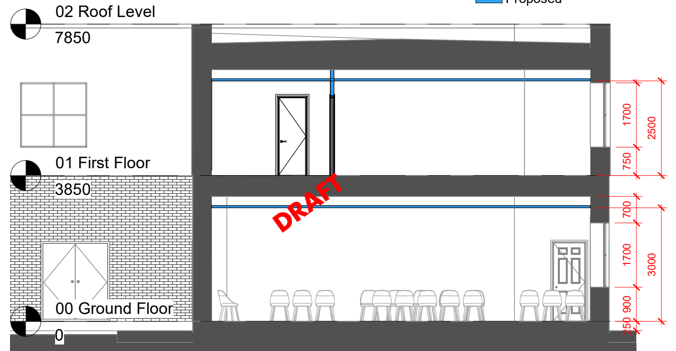
3 Section CC 1 : 100
