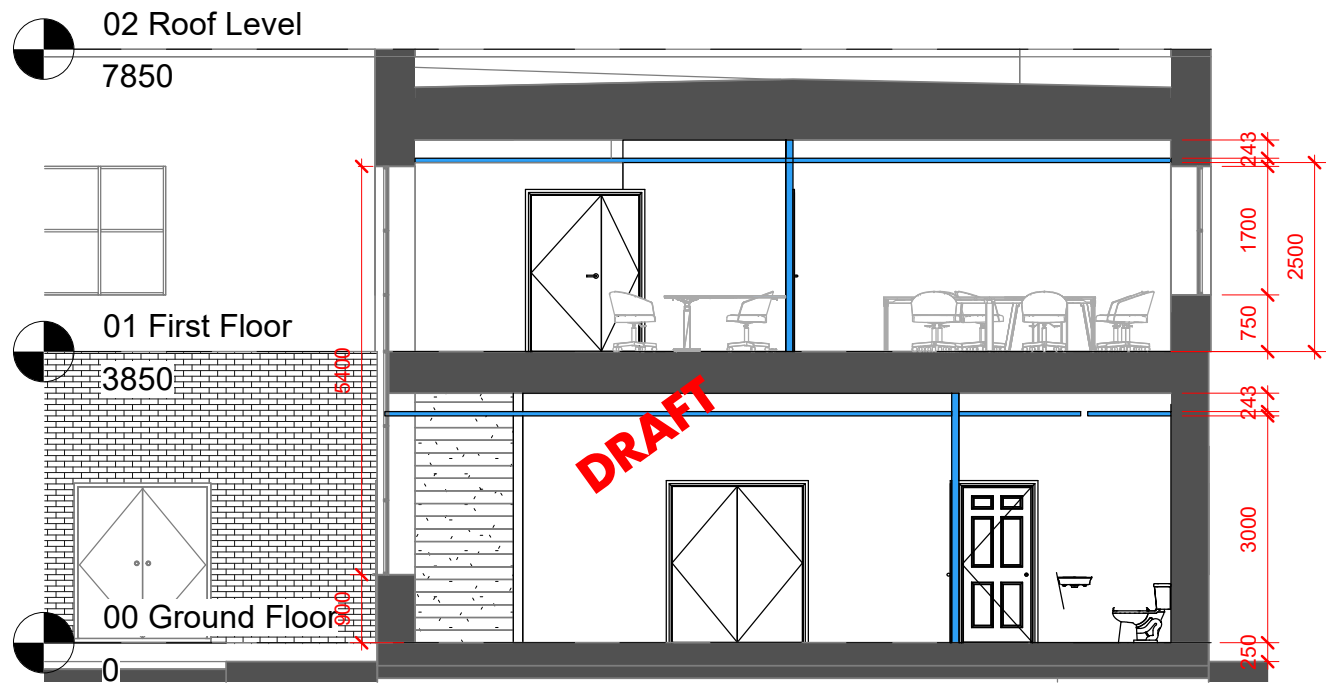
2 Section BB 1 : 100
