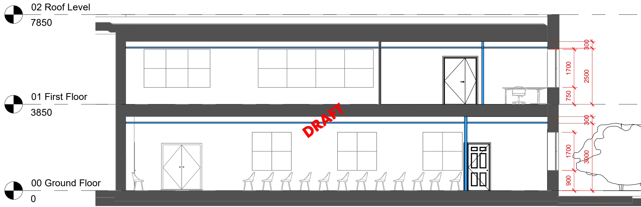
1 Section AA 1 : 100
